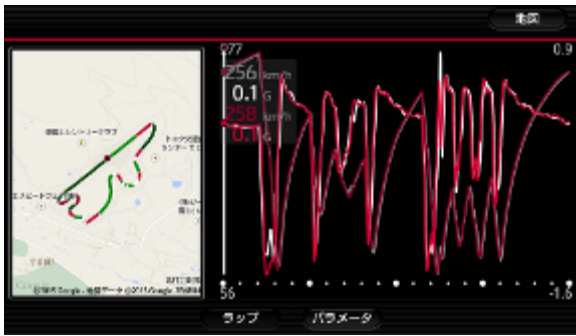
走行ライン図・車速・前後G表示例
