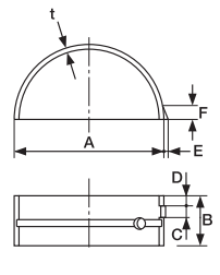
メインベアリング
