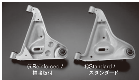
⑤Rear A Arm / リアアーム
