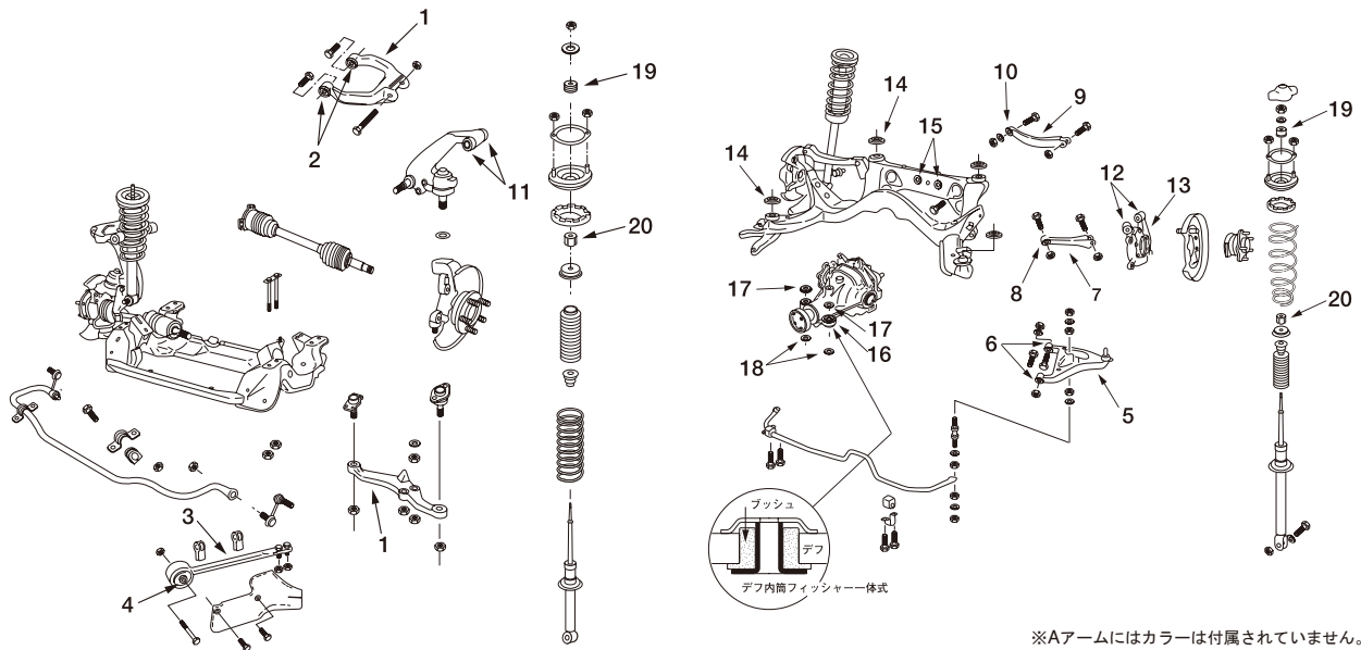
⑤Rear A Arm / リアアーム
